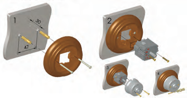
D Con peana Garby en pared Avec socle Garby sur mur With Garby base on wall
