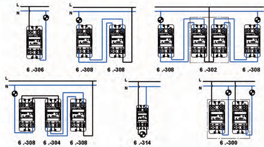
Esquemas de conexión Venezia/ F-37 Schèmes de connexion Venezia/ F-37 Venezia/ F-37 connection schemes
