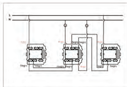
Doble conmutador Double two-way switch
