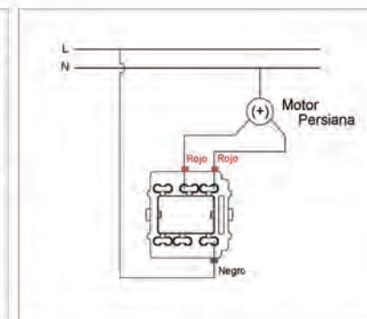
Mecanismos para persianas Electric blinds mechanism
